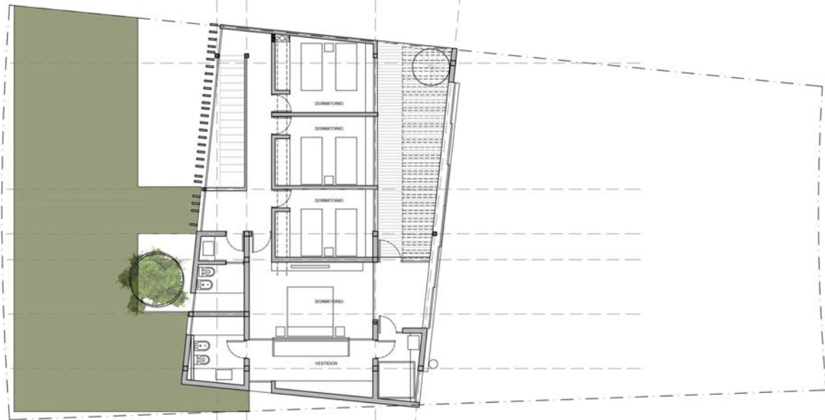
PLANTA ALTA
